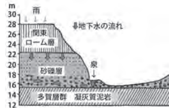
泉が森の湧水模式図 (出典:『日立の湧水』)
